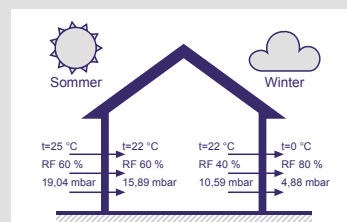
Transport wilgoci i różnica ciśnień
