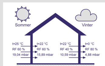
Fugtens vandring sommer/vinter
