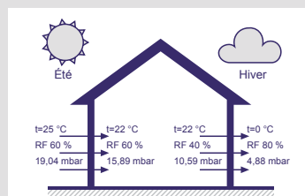
Transport d'humidité et différence de pression
